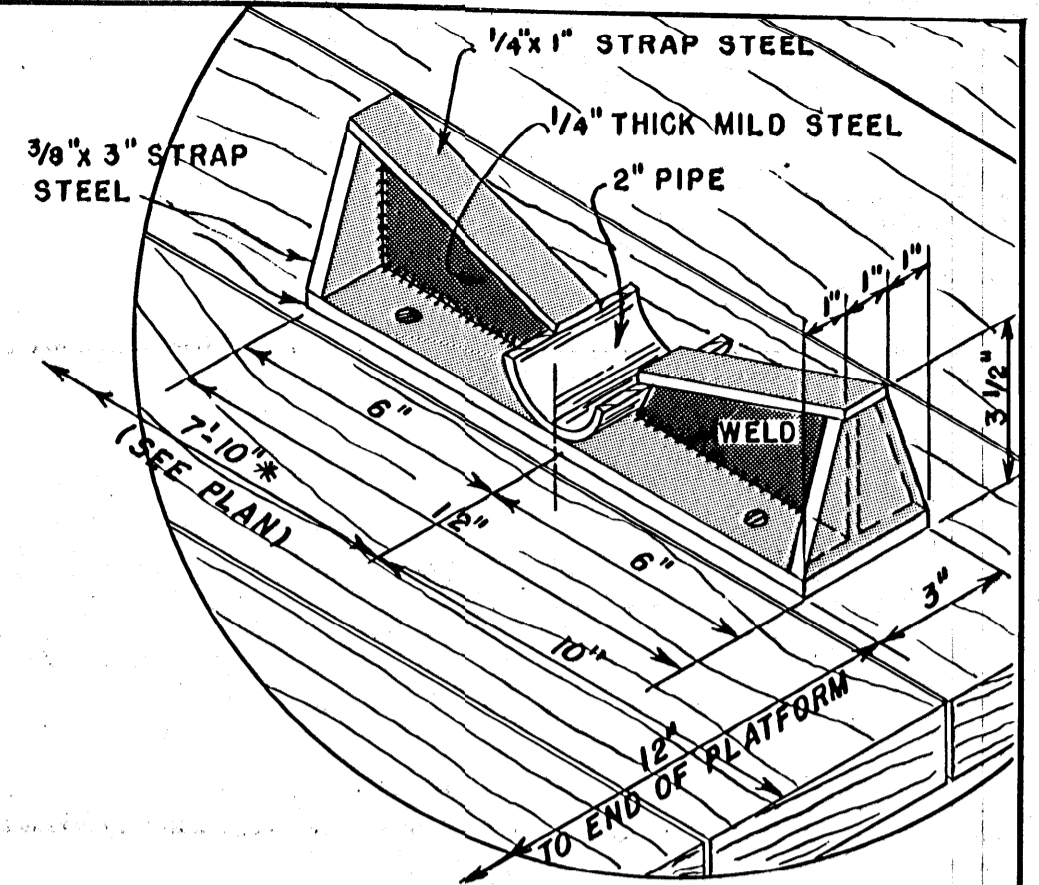
DETAIL "B" SCALE: 3" = 1'-0"
